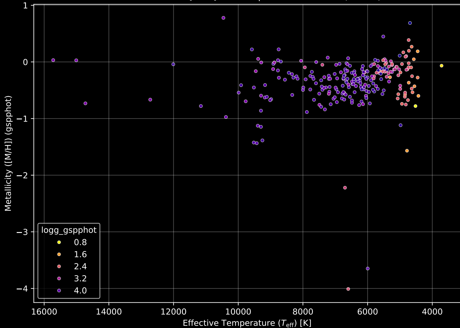
GALAH DR4 Field: [9400] Stellar Population Parameters (n= 253)
