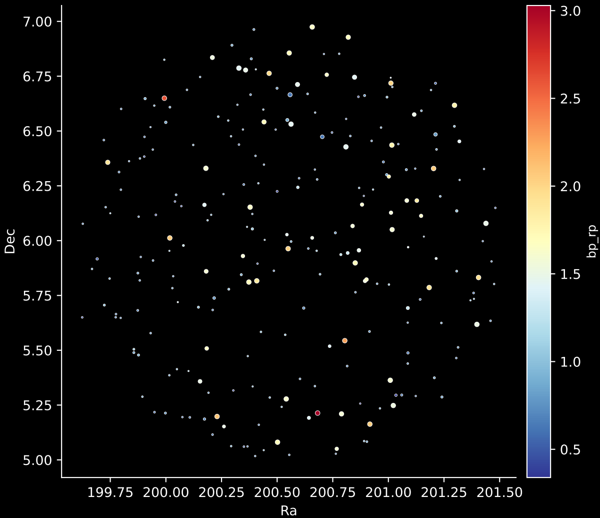
GALAH DR4 Field: [9400] Stars: 253
