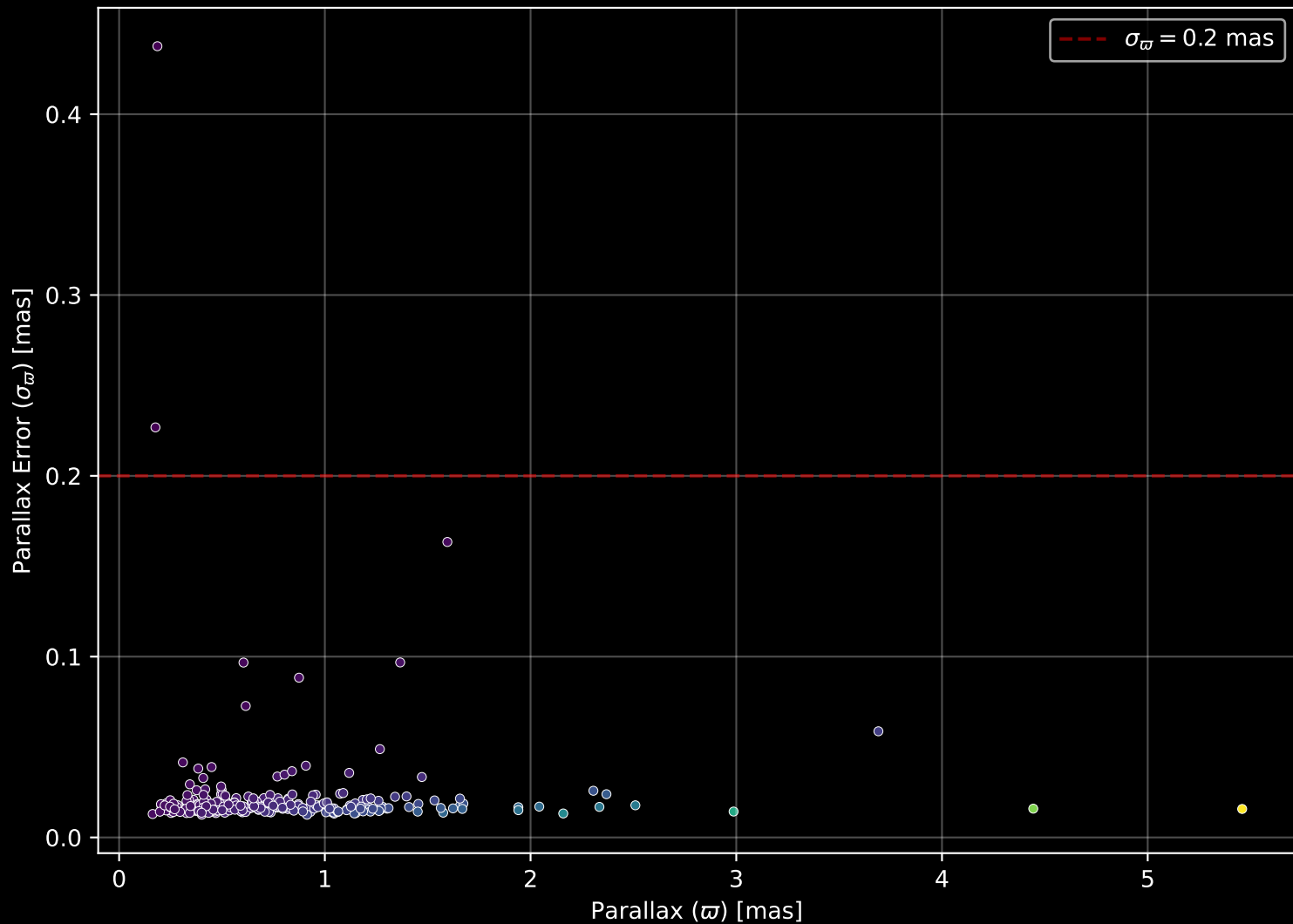
GALAH DR4 Field: [9400] Parallax Quality (n= 253)
