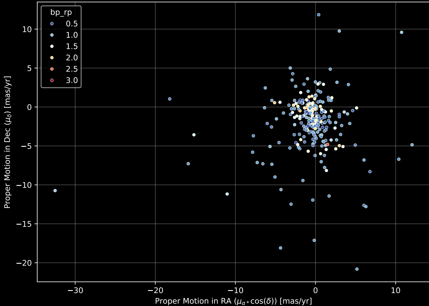
GALAH DR4 Field: [9400] Proper Motion Diagram (n= 253)
