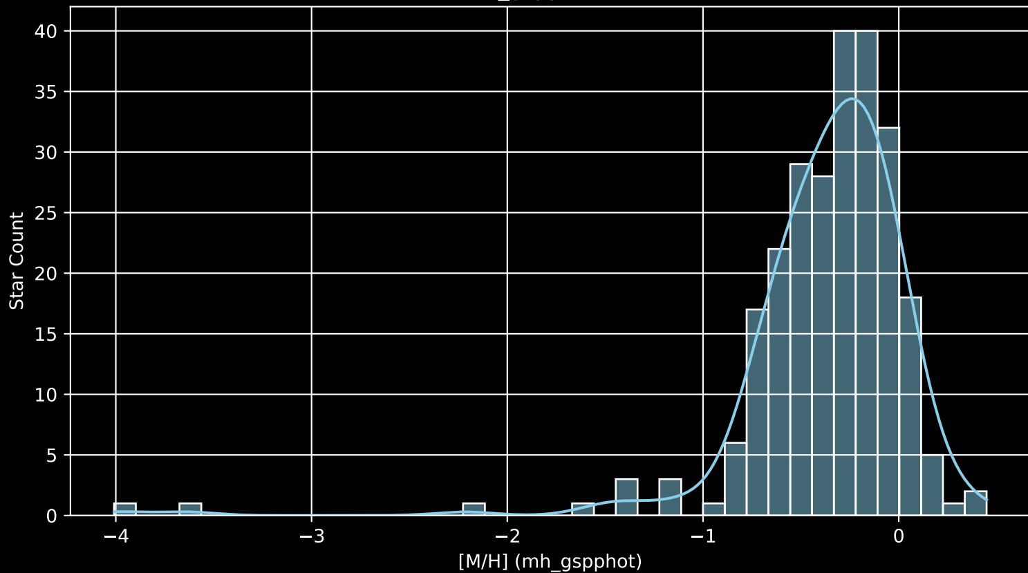
GALAH DR4 Field: [9400] [M/H] (mh_gspphot) (n= 251)
